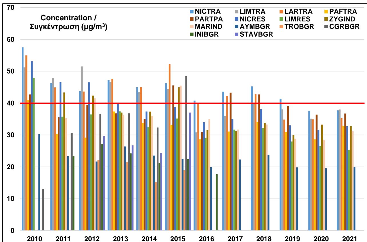
Σχήμα 11: Ετήσιοι μέσοι όροι ΑΣ 10 στους Σταθμούς Παρακολούθησης Ποιότητας Αέρα για την περίοδο 2010-2021 (Ετήσια οριακή τιμή: 40 µg/m 3 ).
