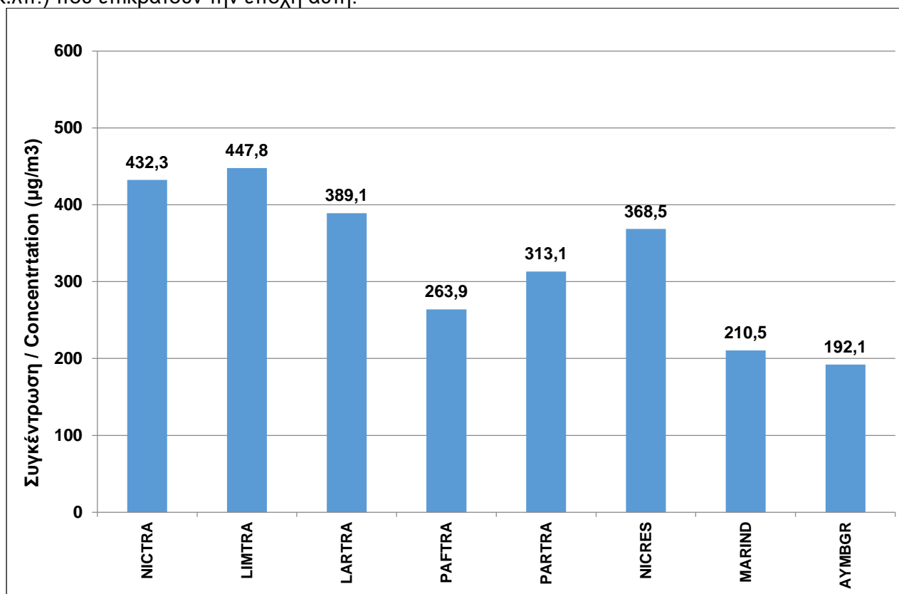
Σχήμα 9: Ετήσιοι μέσοι όροι CO στους Σταθμούς Παρακολούθησης Ποιότητας Αέρα για το έτος 2021. Figure 9: CO annual mean concentration in Air Quality Monitoring Stations for the year 2021.
