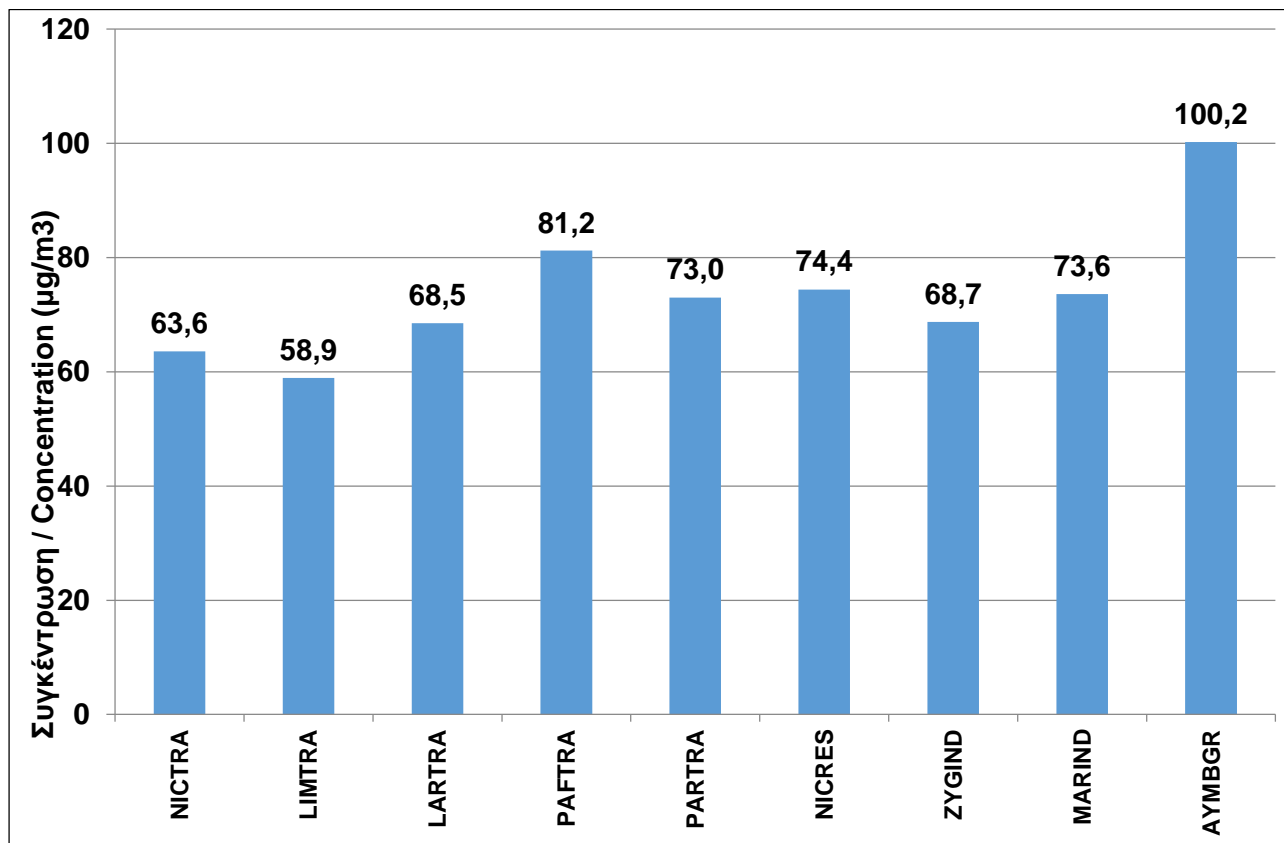
Σχήμα 7: Ετήσιοι μέσοι όροι \text{O}_3 στους Σταθμούς Παρακολούθησης Ποιότητας Αέρα για το έτος 2021. Figure 7: \text{O}_3 annual mean concentration in Air Quality Monitoring Stations – for the year 2021.
