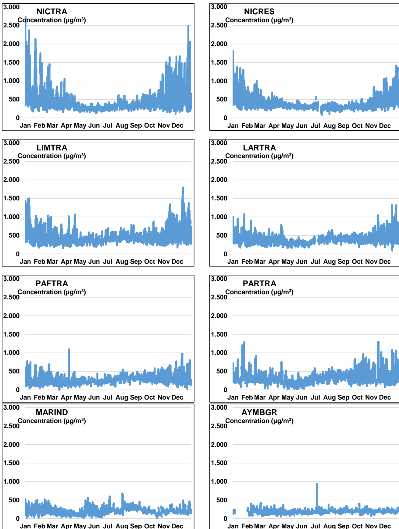
Σχήμα 10: Μέσες 8-ωρες τιμές μονοξειδίου του άνθρακα (CO) στους Σταθμούς Παρακολούθησης Ποιότητας Αέρα για το έτος 2021 (Οριακή Τιμή μέγιστου ημερήσιου μέσου όρου οκταώρου: 10.000 µg/m³).
