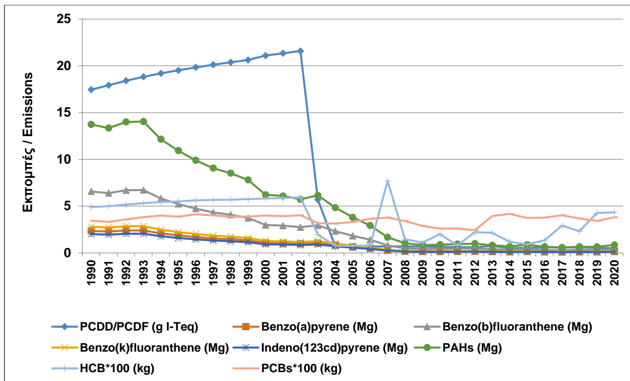
Σχήμα 22: Τάσεις εκπομπών για τους Έμμοτους Οργανικούς Ρύπους για την περίοδο 1990-2020.
