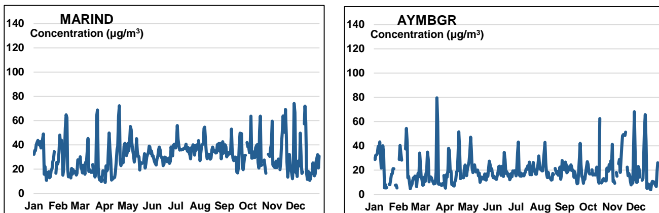
Σχήμα 14: Ημερήσια συγκέντρωση Αιωρούμενων Σωματιδίων με αεροδυναμική διάμετρο 10 µm (ΑΣ 10 ) στους Σταθμούς Παρακολούθησης Ποιότητας Αέρα για το έτος 2021 (Ημερήσια οριακή τιμή: 50 µg/m 3 ).
