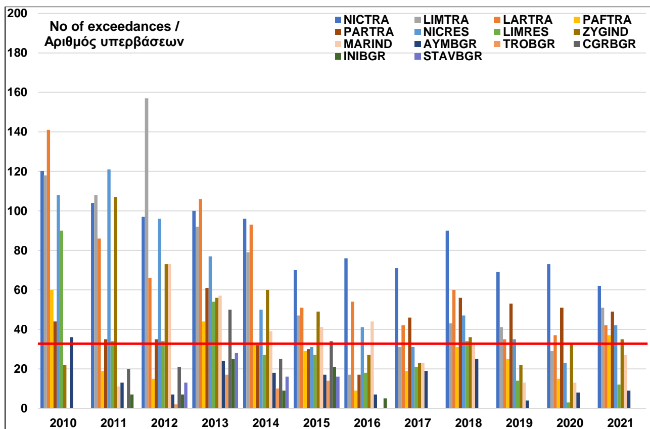
Σχήμα 12: Αριθμός υπερβάσεων ανά έτος της ημερήσιας οριακής τιμής ΑΣ 10 στους Σταθμούς Παρακολούθησης Ποιότητας Αέρα για την περίοδο 2010-2021 (Αριθμός επιτρεπτών υπερβάσεων: 35).
