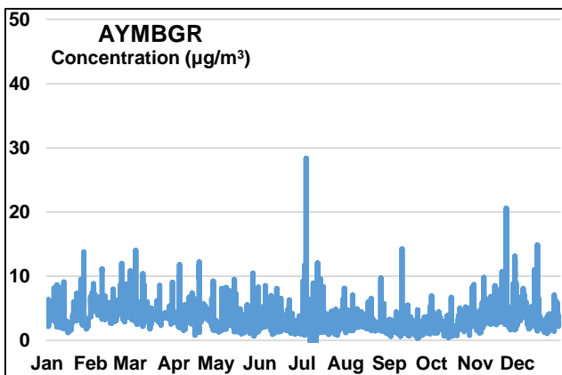
Σχήμα 5: Μέσες ωριαίες τιμές διοξειδίου του αζώτου ( \text{NO}_2 ) στους Σταθμούς Παρακολούθησης Ποιότητας Αέρα για το έτος 2021 (Ωριαία οριακή τιμή: 200 \mu\text{g}/\text{m}^3 ).
