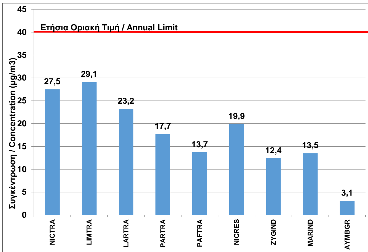
Σχήμα 4: Ετήσιοι μέσοι όροι \text{NO}_2 στους Σταθμούς Παρακολούθησης Ποιότητας Αέρα για το έτος 2021. Figure 4: \text{NO}_2 annual mean concentration in Air Quality Monitoring Stations for the year 2021.
