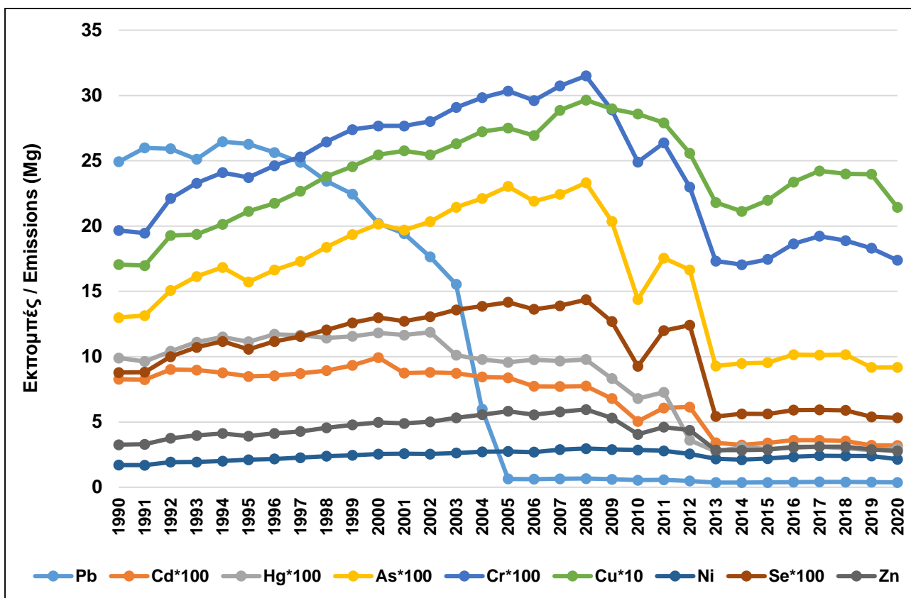
Σχήμα 21: Τάσεις εκπομπών για τα βαρέα μέταλλα για την περίοδο 1990-2020. Figure 21: Emission trends for heavy metals for the period 1990-2020.
