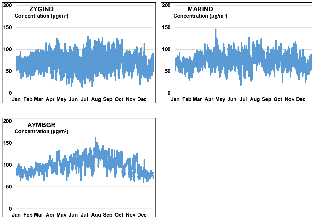
Σχήμα 8: Μέσες 8-ωρες τιμές όζοντος ( O_3 ) στους Σταθμούς Παρακολούθησης Ποιότητας Αέρα για το έτος 2021 (Μέγιστος ημερήσιος μέσος όρος οκταώρου – Τιμή Στόχος: 120 \mu\text{g}/\text{m}^3 ).
