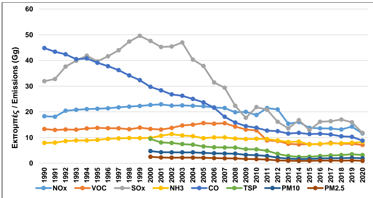
Σχήμα 20: Τάσεις εκπομπών για τους κύριους ρύπους και τα σωματίδια για την περίοδο 1990-2020. Figure 20: Emission trends for main pollutants and particulates for the period 1990-2020.
