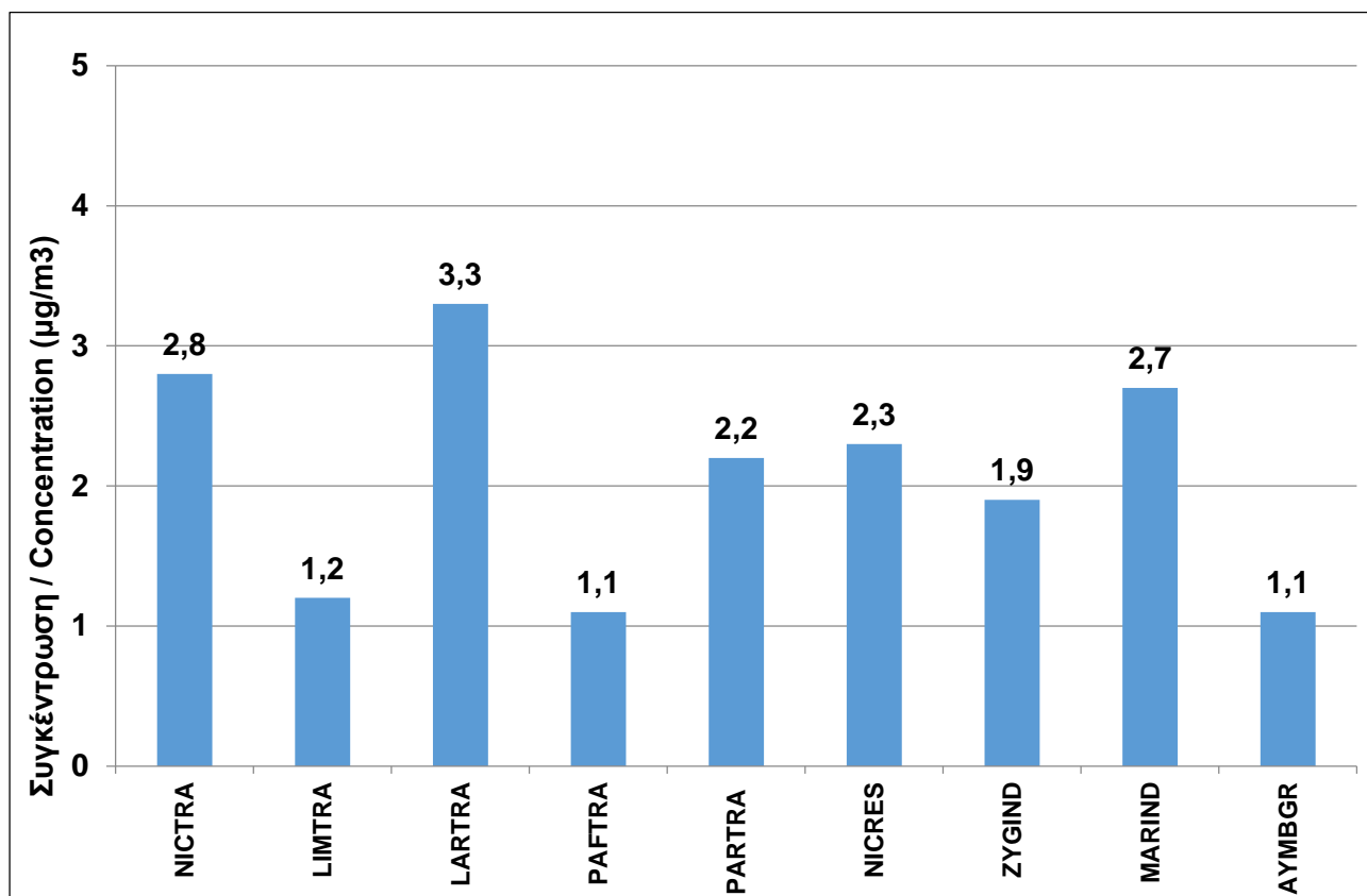
Σχήμα 6: Ετήσιοι μέσοι όροι \text{SO}_2 στους Σταθμούς Παρακολούθησης Ποιότητας Αέρα για το έτος 2021. Figure 6: \text{SO}_2 annual mean concentration in Air Quality Monitoring Stations for the year 2021.
